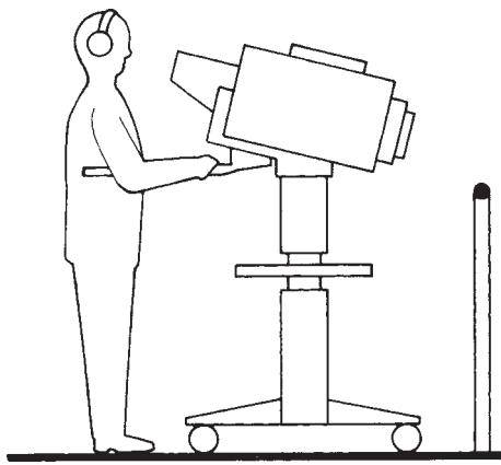
Позиция телеоператора. Минимальные размеры площадки: 1,5 x 1,0 м.
